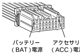
ホンダ車用の20ピンコネクターの例
