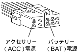
日産車用の10ピンコネクターの例（'93.8以前）
