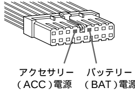
ホンダ車用の16ピンコネクターの例
