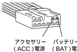
トヨタ車用の10ピンコネクターの例
