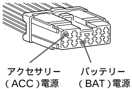
日産車用の10ピンコネクターの例（'93.8以降）
